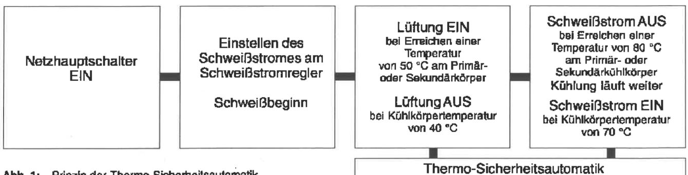
Abb. 1: Prinzip der Thermo-Sicherheitsautomatik
