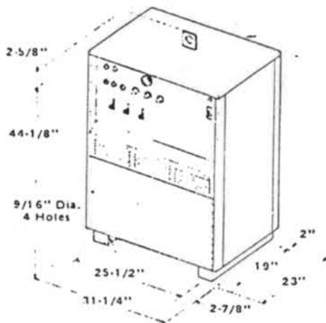
Fig. 3-1 Dimensionen
