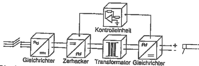
Bild 3 - Blockdiagramm eines Inverter-Schweißgleichrichters (Umrichter)
