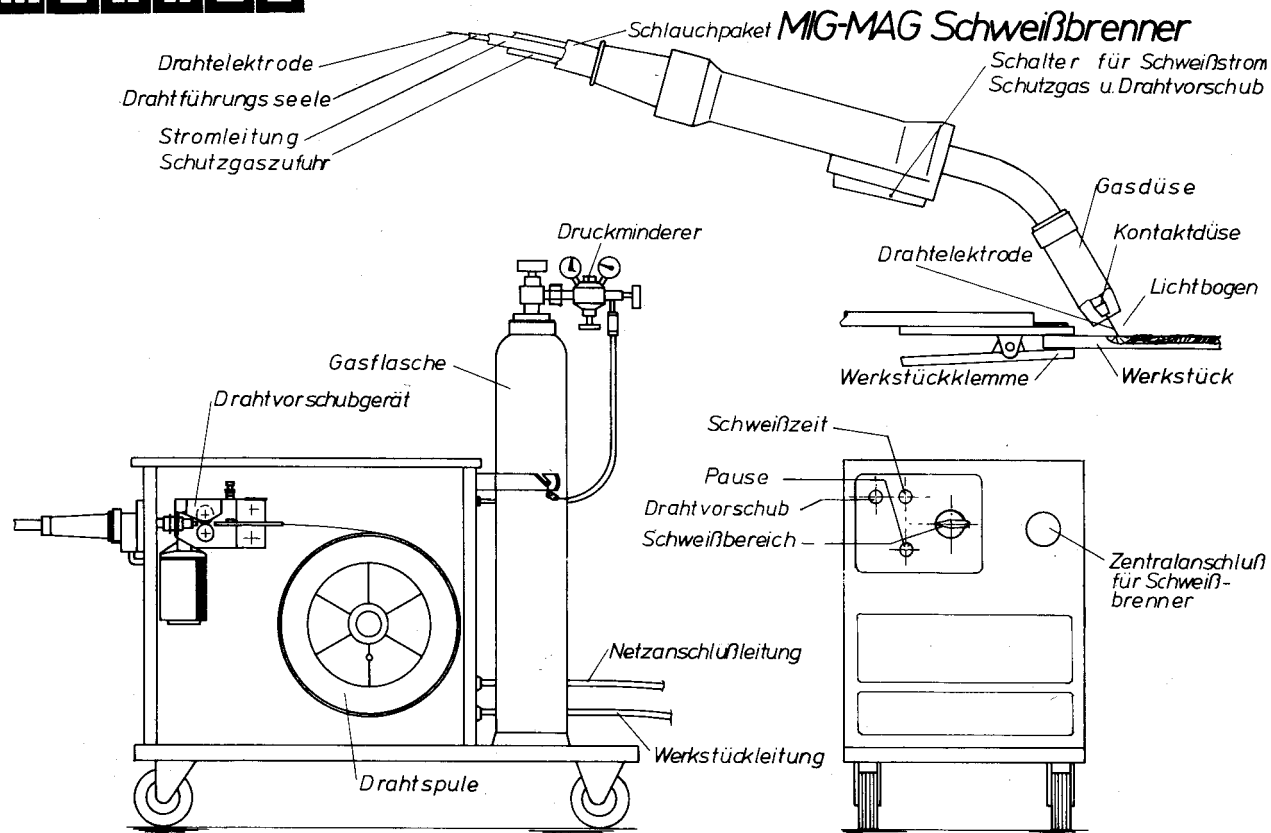
MIG-MAG Schutzgasschweißanlage
