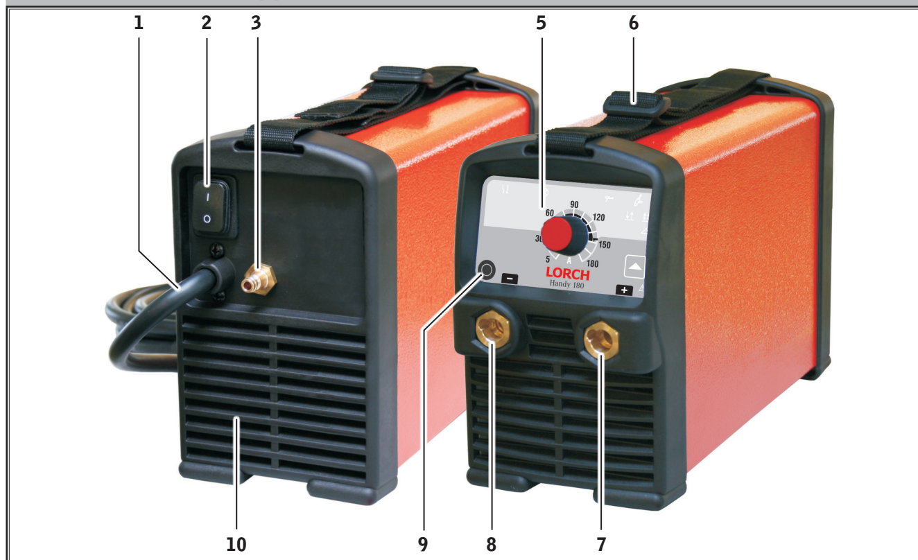
Fig. 11: Éléments de l'appareil
