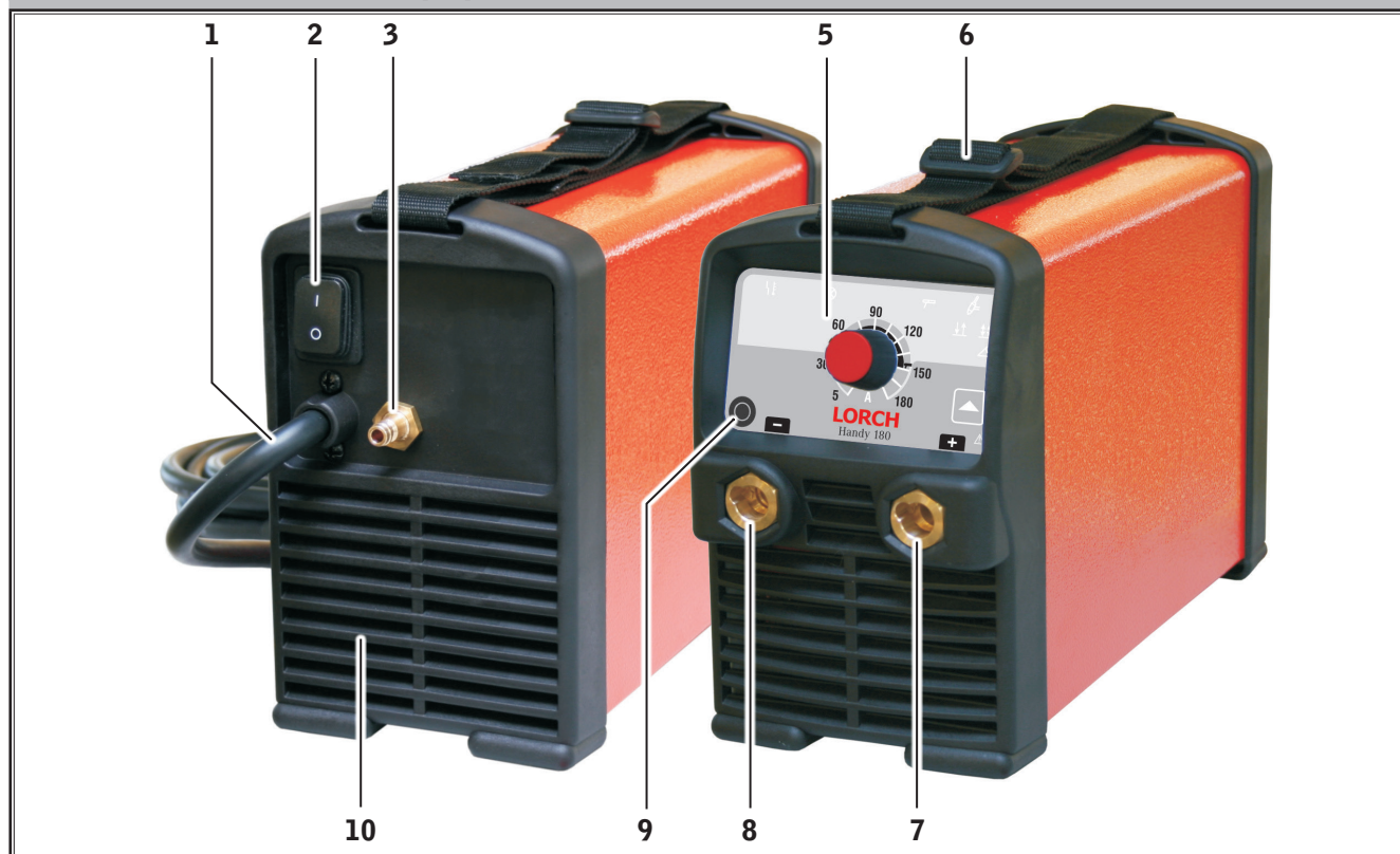
Abb. 1: Elementos del equipo
