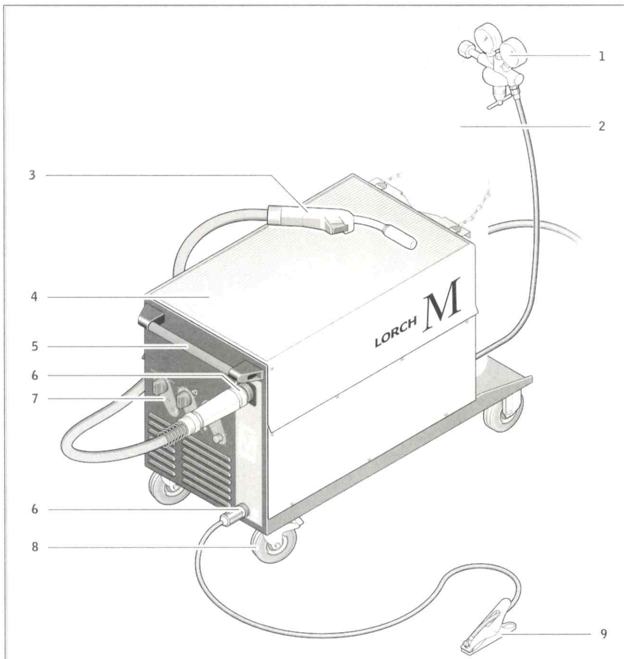
Abb. 1: Geräteelemente
