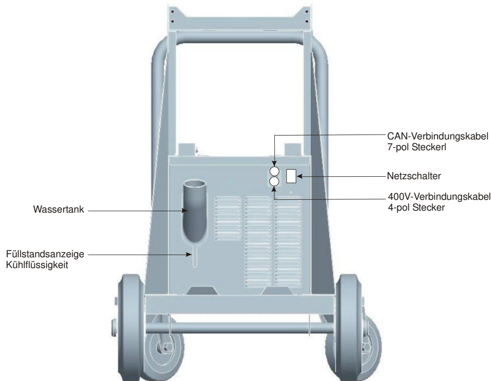
Bild 3: TIG - COOL CART 2000 Ansicht von Hinten
