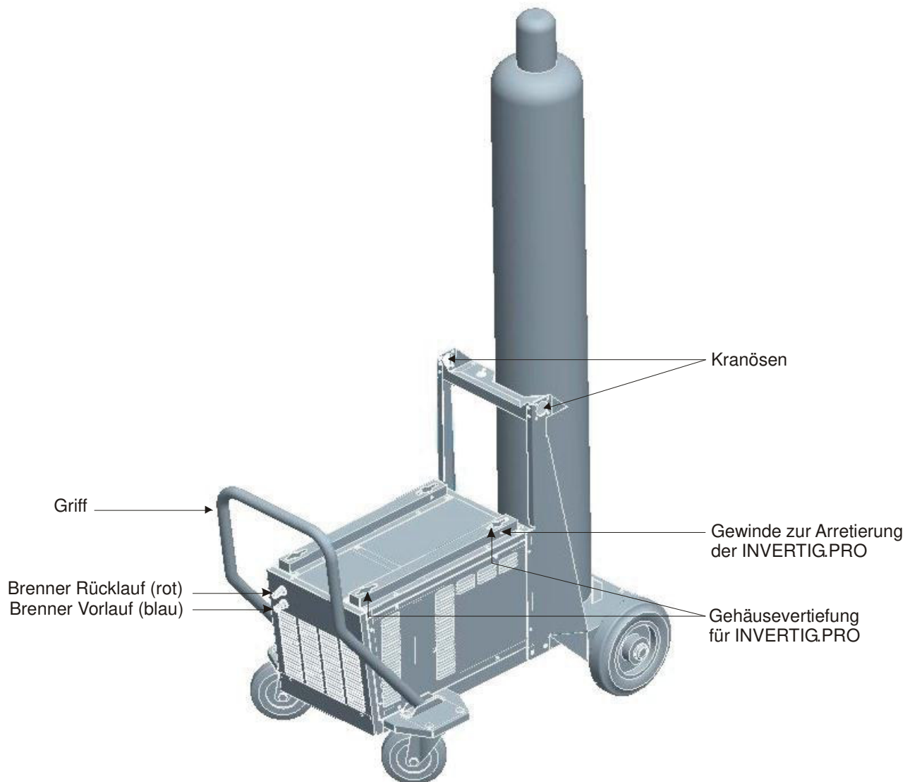
Bild 2: TIG – COOL CART 2000 mit Gasflasche
