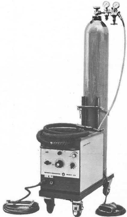
Bild 2 MIGBOY 200 mit Fahrwagen
