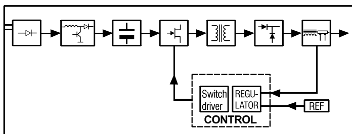
DELTA 180E PFC blokkdiagram
